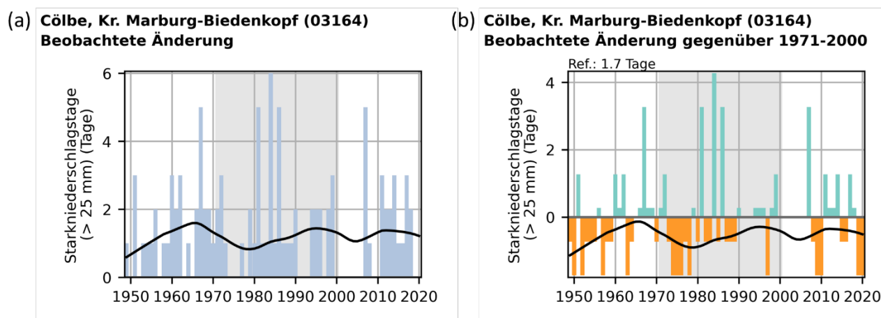
Abbildung 45: Dargestellt ist die beobachtete Änderung der Starkniederschlagstage (a) als absoluter Wert und (b) als Anomalie gegenüber der Referenzperiode 1971–2000 an der DWD-Station Cölbe, Kr. Marburg-Biedenkopf (03164).
