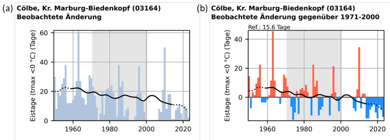
Abbildung 42: Dargestellt ist die beobachtete Änderung der Eistage (a) als absoluter Wert und (b) als Anomalie gegenüber der Referenzperiode 1971—2000 an der DWD-Station Cölbe, Kr. Marburg-Biedenkopf (03164).
