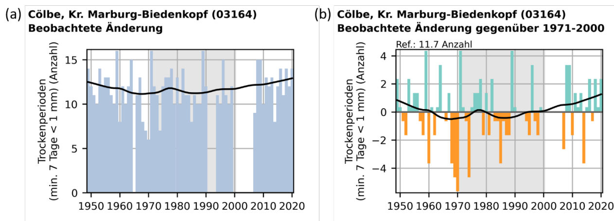
Abbildung 46: Dargestellt ist die beobachtete Änderung der Trockenperioden (a) als absoluter Wert und (b) als Anomalie gegenüber der Referenzperiode 1971–2000 an der DWD-Station Cölbe, Kr. Marburg-Biedenkopf (03164).
