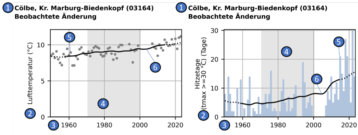
Abbildung 35: Beschreibung und Legende zur absoluten Darstellung der Klimaindizes: 1. Übergeordneter Titel: Plot zeigt beobachtete Daten an der angegebenen Station. Datengrundlage sind DWD-Stationsdaten. 2. Klimaindex: Y-Achse zeigt die Werte des Klimaindex mit der dazugehörigen Skala. 3. Zeithorizont: X-Achse zeigt die zeitliche Dimension der dargestellten Klimaindizes. 4. Referenzbereich: Grau hinterlegter Bereich zeigt die Referenzperiode (1971–2000) für die Berechnung der Anomalie. 5. Jahreswert: Jeder Punkt (oder Balken) zeigt den aggregierten Jahresmittel- oder Jahressummenwert. 6. Trendlinie: Geglättetes 20-jähriges Mittel der aggregierten Jahreswerte. Die gepunkteten Randbereiche (jeweils 10 Jahre) zeigen den unsicheren Bereich der Trendlinie. Bei den niederschlagsbezogenen Indizes zeigt die Trendlinie den LOESS-Filter und repräsentiert das 30-jährige Mittel der aggregierten Jahreswerte.
